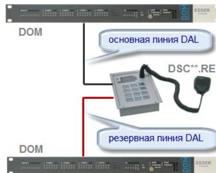
Рисунок 15 –Резервное подключение консоли
