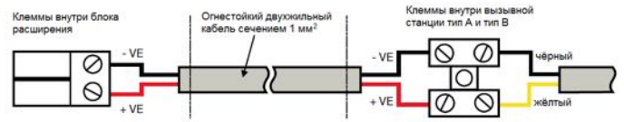
Рисунок 94 – Схема подключения вызывных станций к блоку связи (расширения)
