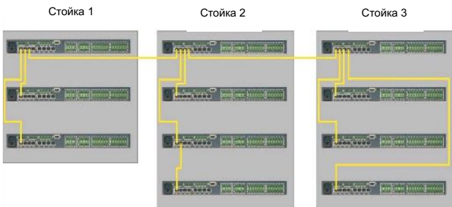
Рисунок 33 Пример распределённого подключения стоек (сетевое оборудование ЛВС не показано)
