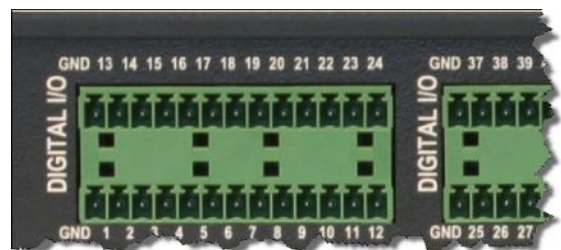
Рисунок 20 – Контактные группы модуля UIM
