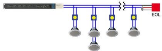
Рисунок 63 - Использование линейных аттенюаторов
