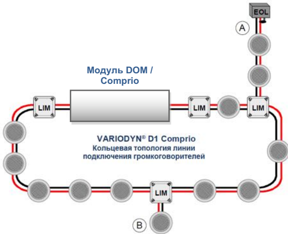
Рисунок 65 - Организация кольцевого шлейфа
