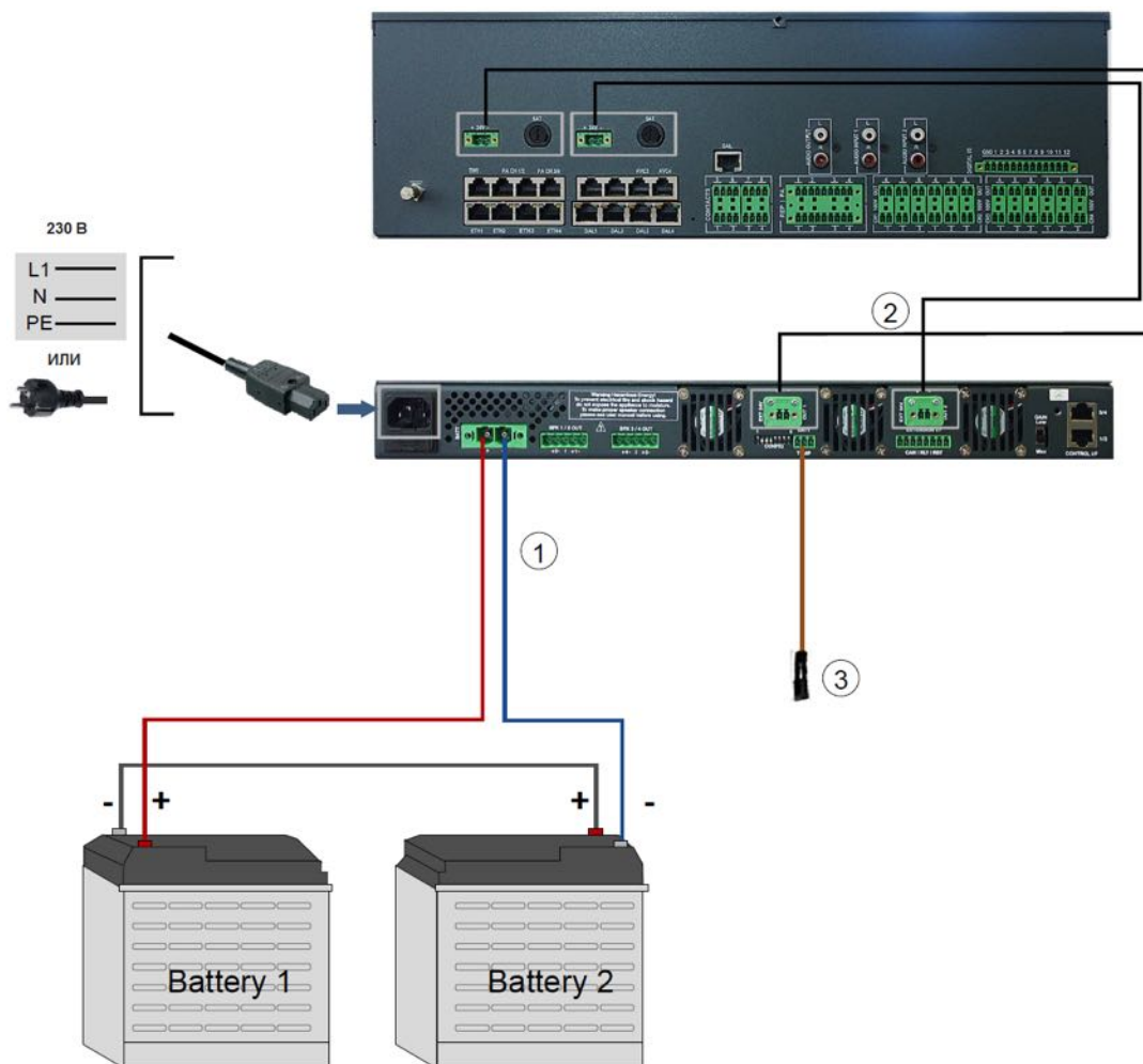
Рисунок 38 – Подключения Comprio и усилителя 4x 125 Вт - питание
