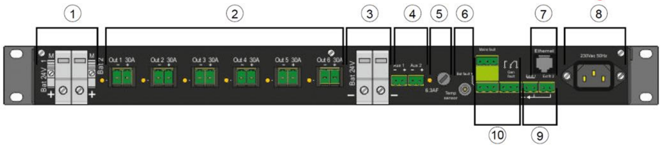
Рисунок 51 – Тыльная сторона ИБП арт. №581722
