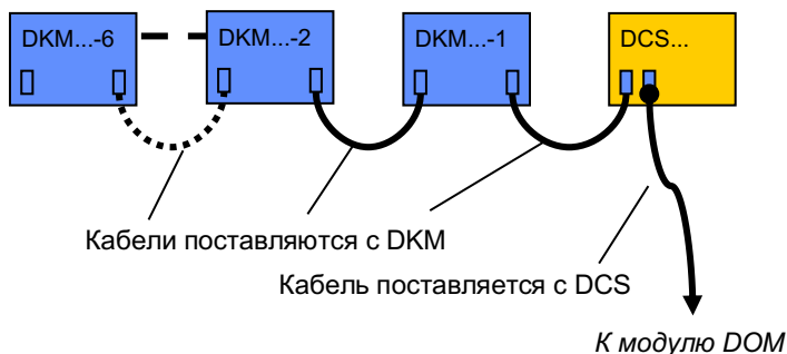
Рисунок 14 – Подключение модулей DKM
