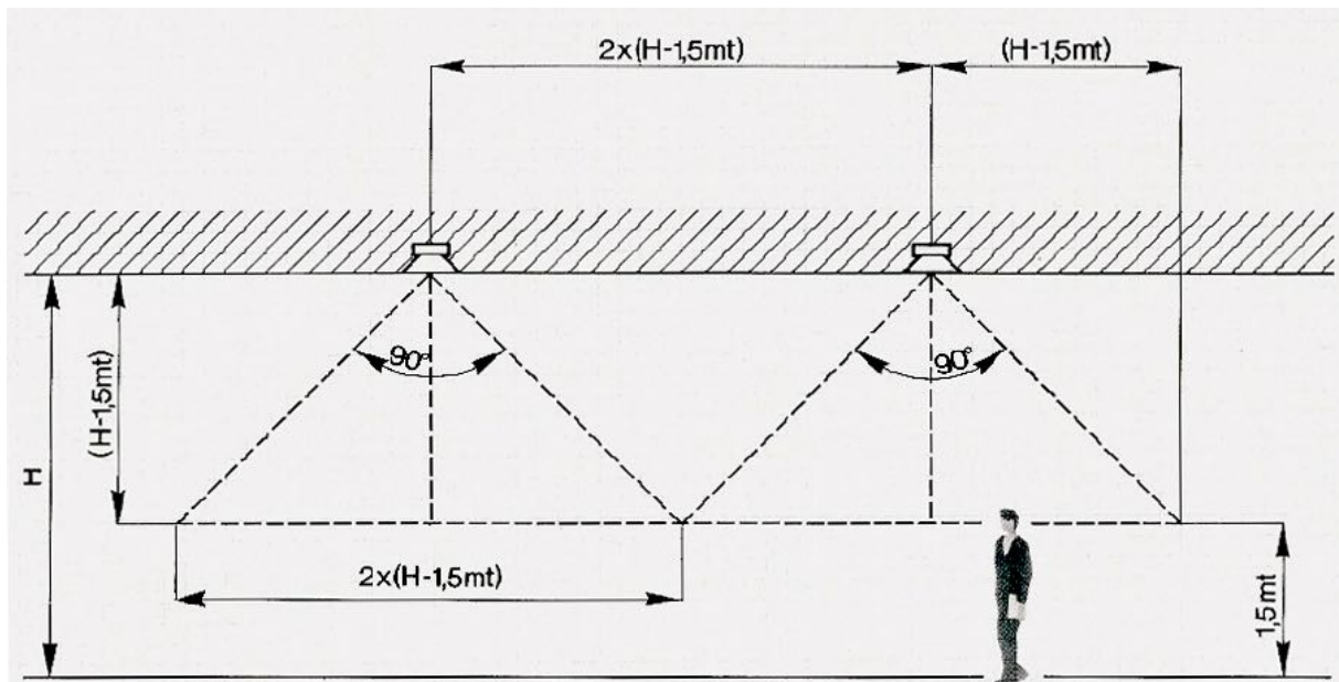
Рисунок 79 - Расчёт расстояния между осями потолочных громкоговорителей
