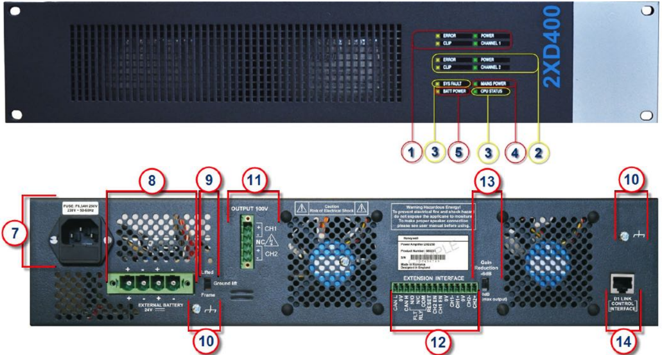
Рисунок 26 – Лицевая и задняя панели двухканального усилителя мощности Variodyn (класс D)
