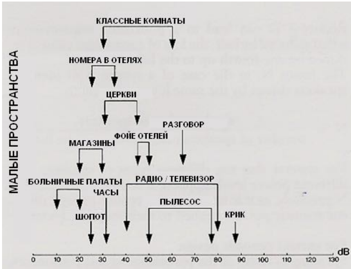
Рисунок 71 - Уровень фонового шума для малых пространств
