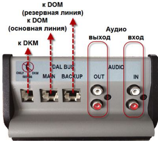
Рисунок 16 – Тыльная сторона консоли DCS15 (арт. № 583501.RE) с резервной линией подключения
