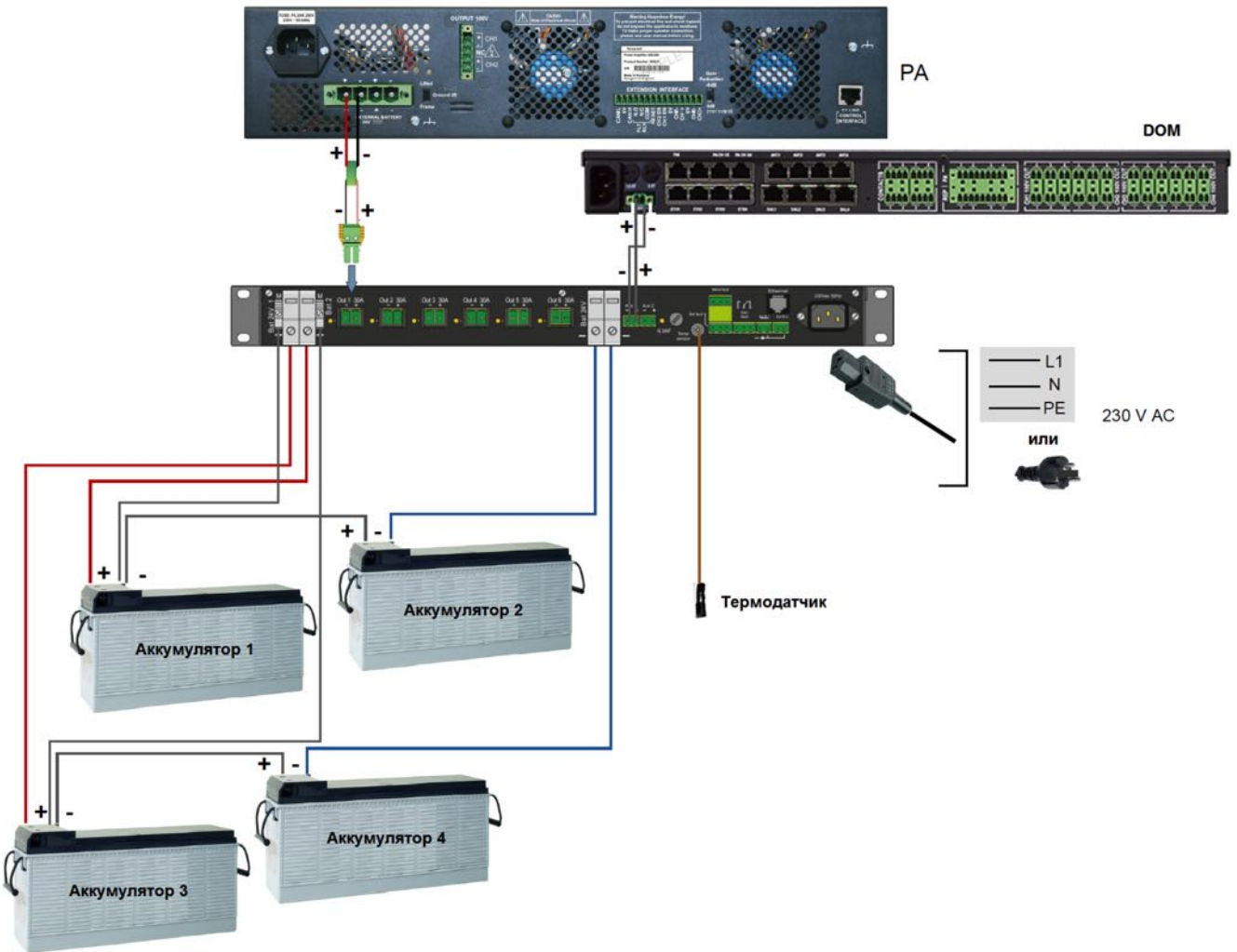
Рисунок 54 – Пример подключения ИБП арт. №581722 с линией выравнивания потенциалов
