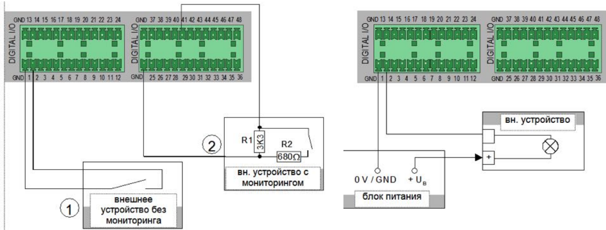
Рисунок 39 – Подключение контактных сигналов (слева – входных, справа – выходных) на модулях UIM и Compro
