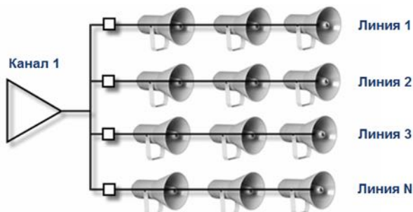
Рисунок 57 – Мультилинейная схема подключения
