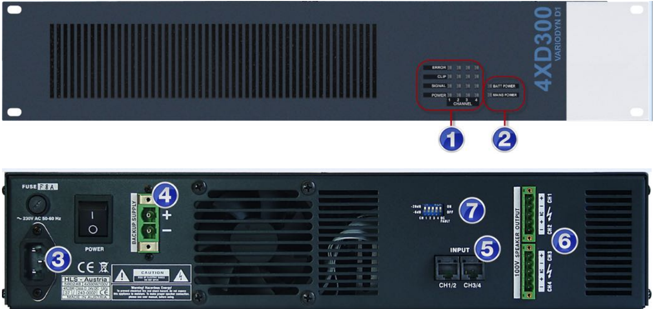
Рисунок 29 – Лицевая и задняя панели четырёхканального усилителя мощности Variodyn (класс D)
