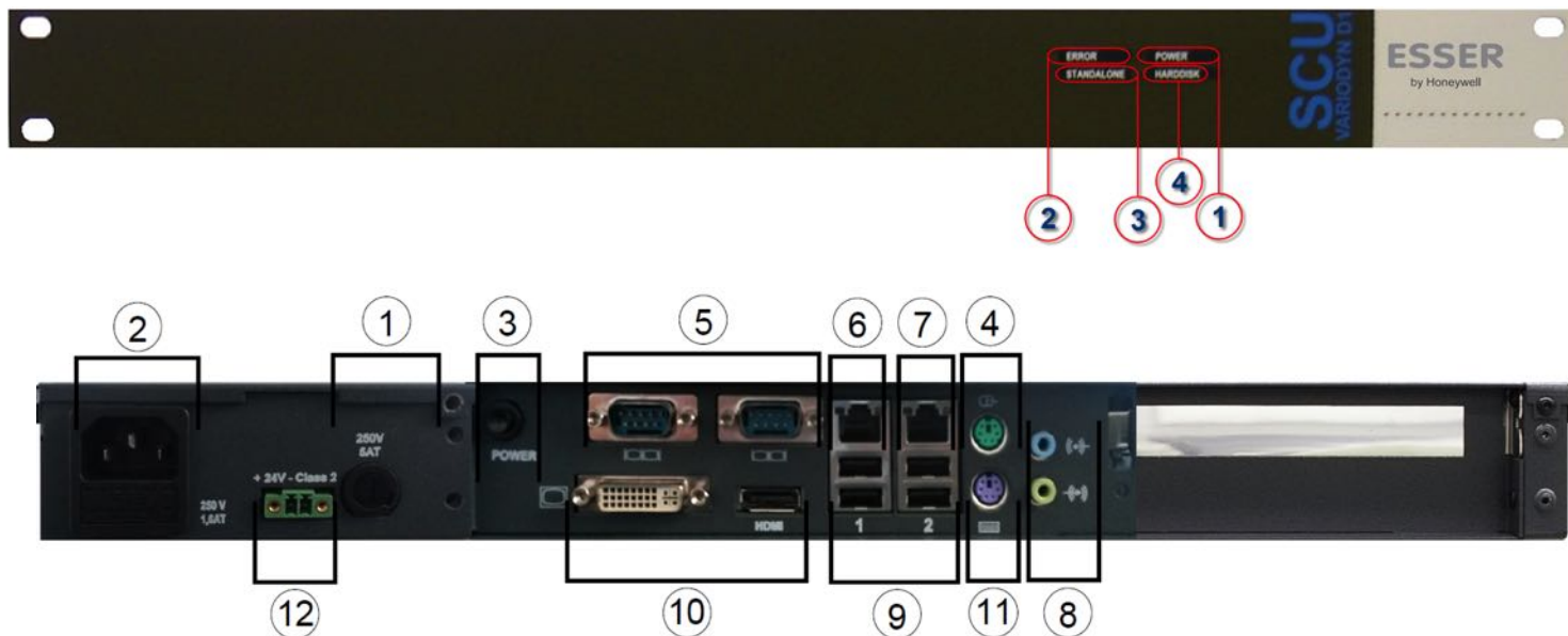
Рисунок 31 – Задняя панель модуля SCU (арт.№ 583381.31)
