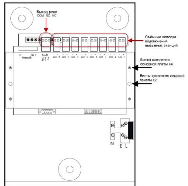
Рисунок 96 – Расположение клемм подключения внутри блока связи (расширения)
