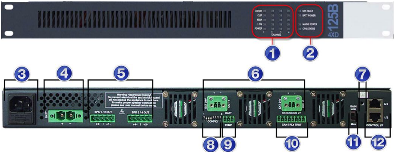
Рисунок 27 – Лицевая и задняя панели четырёхканального усилителя мощности 4XD125B
