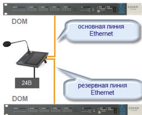
Рисунок 24 – Подключение консоли ETCS
