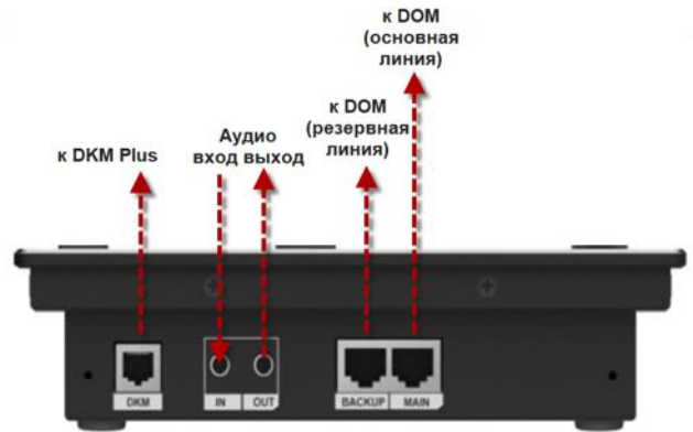
Рисунок 18 – Тыльная сторона консоли DCS Plus (арт. № 583520) с резервной линией подключения
