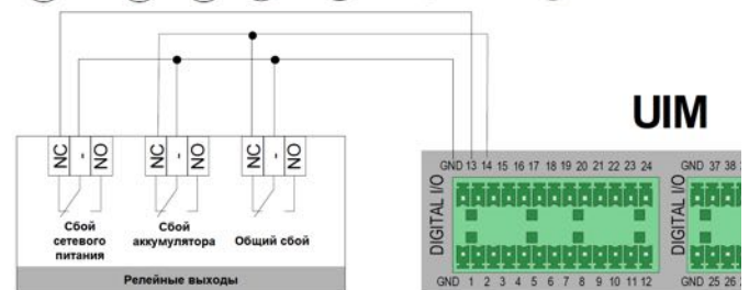
Рисунок 53 – Пример подключения реле неисправности ИБП к модулю UIM
