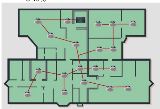
Рисунок 59 - Пример А: Линия оповещения на 20 громкоговорителей
