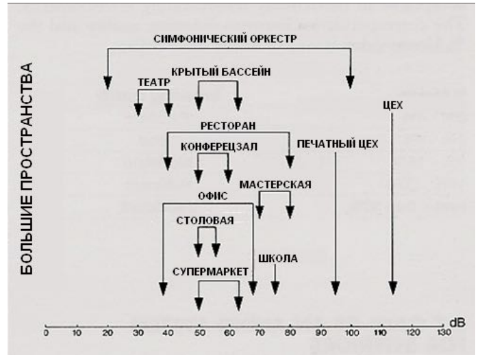
Рисунок 72 - Уровень фонового шума для больших пространств
