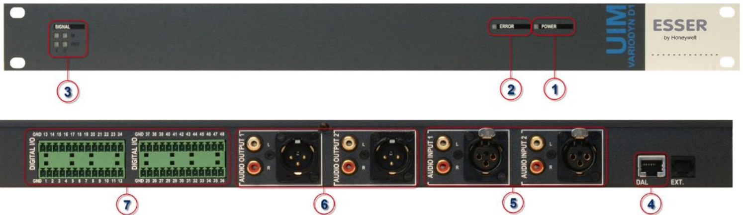
Рисунок 19 – Лицевая и задняя панели модуля UIM
