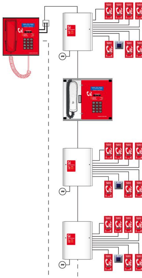
Рисунок 87 – топология системы VoCall
