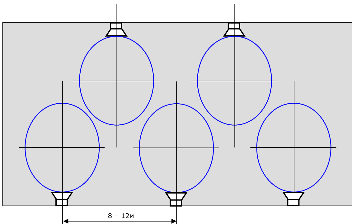
Рисунок 77 - Схема расположения громкоговорителей для помещений шириной более 6 м
