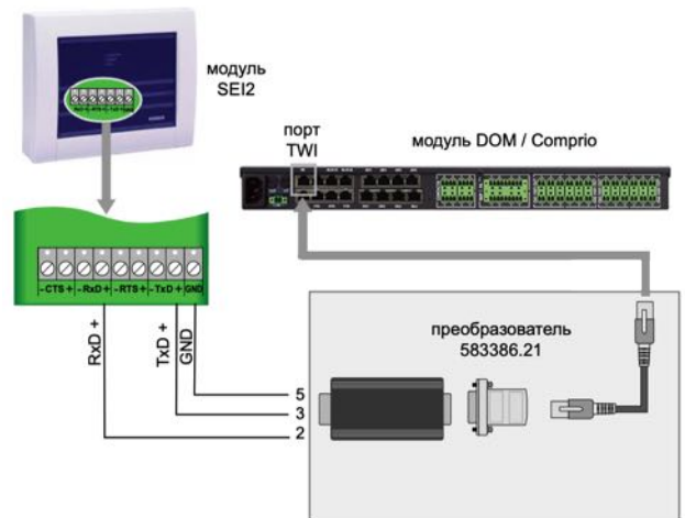
Рисунок 44 – Подключение модуля SEI2
