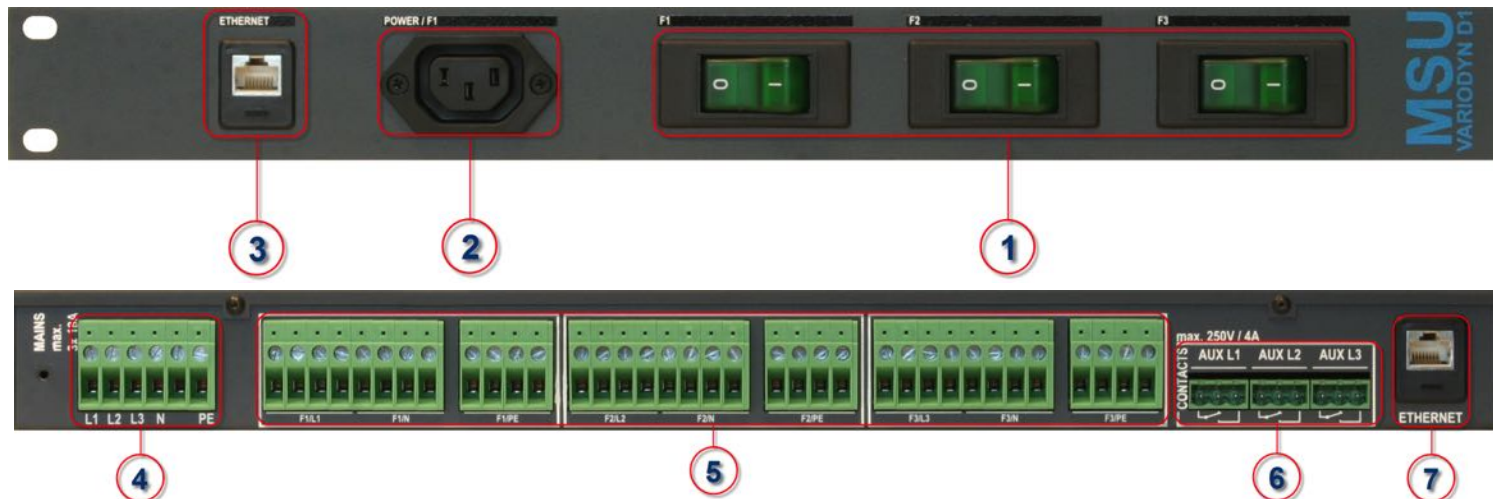
Рисунок 32 – Лицевая и задняя панели модуля MSU
