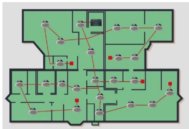
Рисунок 61 - Пример Б: Линия оповещения более 20 громкоговорителей с ответвлениями
