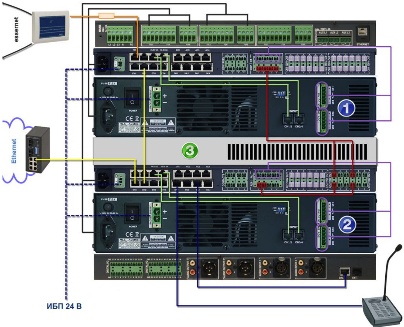
Рисунок 36 – Пример расключения в стойке основных элементов системы (модули DOM, UIM, 4-канальные усилители)
