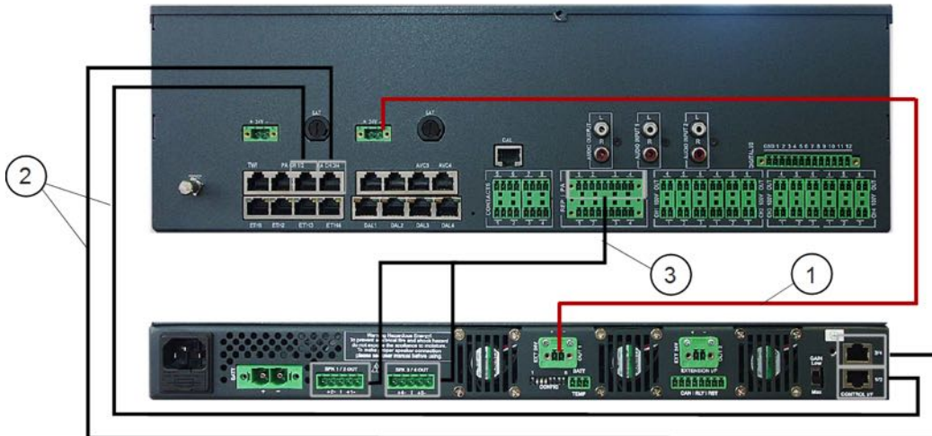
Рисунок 37 – Подключения Comprio и усилителя 4x 125 Вт
