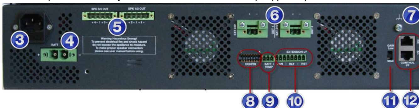
Рисунок 28 – Задняя панель четырёхканального усилителя мощности 4XD250B
