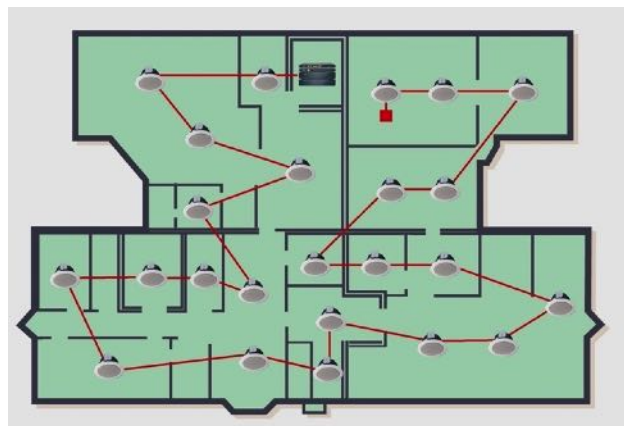
Рисунок 60 - Пример Б: Линия оповещения более 20 громкоговорителей
