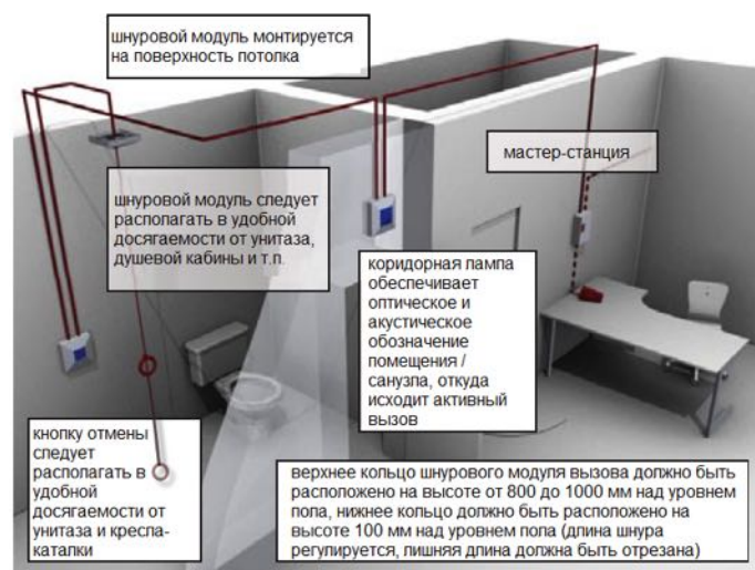
Рисунок 92 – : Рекомендации по размещению вызывного комплекта для МГН
