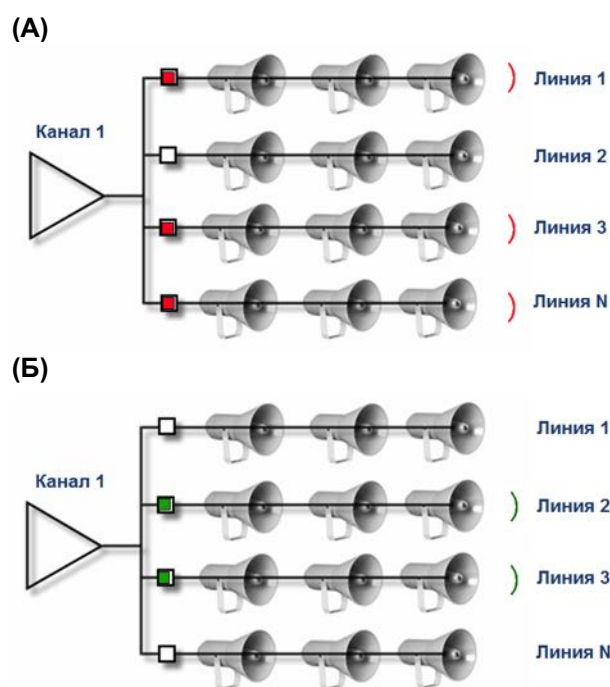
Рисунок 58 - Пример работы мультилинейной схемы
