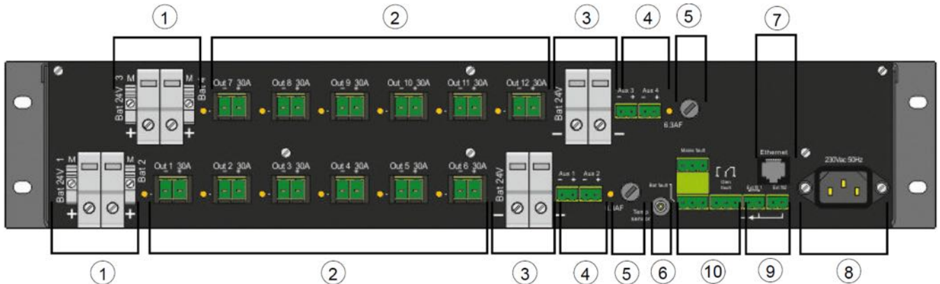
Рисунок 52 – Тыльная сторона ИБП арт. №581723
