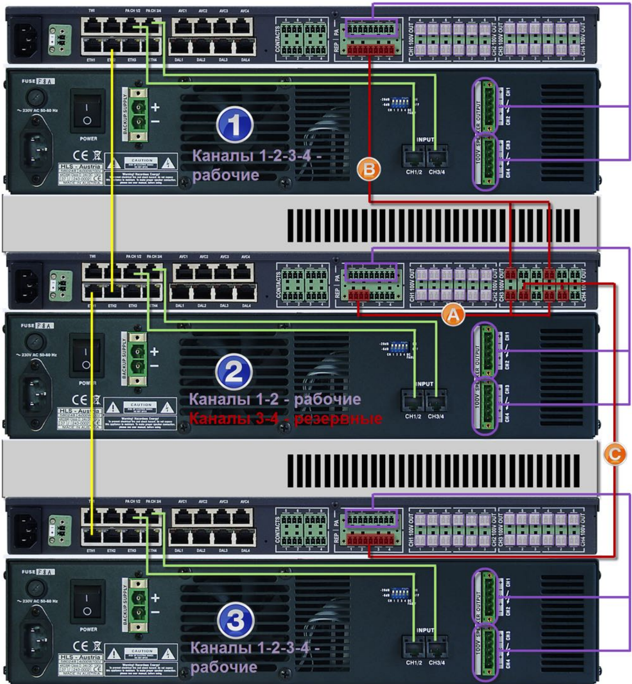
Рисунок 42 – Подключение резервных каналов усиления
