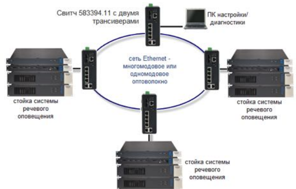
Рисунок 35 Построение кольцевой оптоволоконной сети Ethernet
