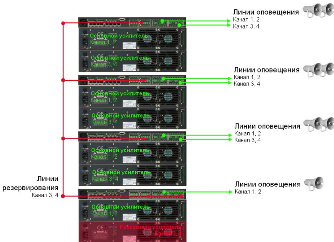
Рисунок 41 – Принцип организации резервных каналов усиления в системе Variodyn D1
