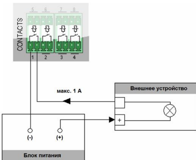
Рисунок 40 – Подключение контактных сигналов (с релейных выходов) на модулях DOM и Compro
