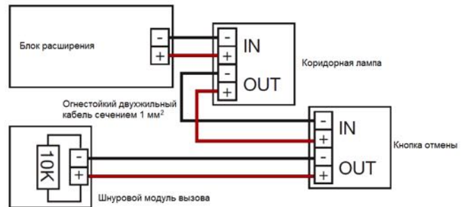
Рисунок 95 – Схема подключения вызывного комплекта для МГН к блоку связи (расширения)
