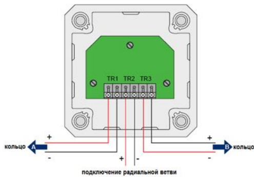
Рисунок 66 - Подключение модуля LIM
