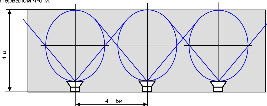
Рисунок 76 - Схема расположения громкоговорителей для помещений шириной менее 6 м
